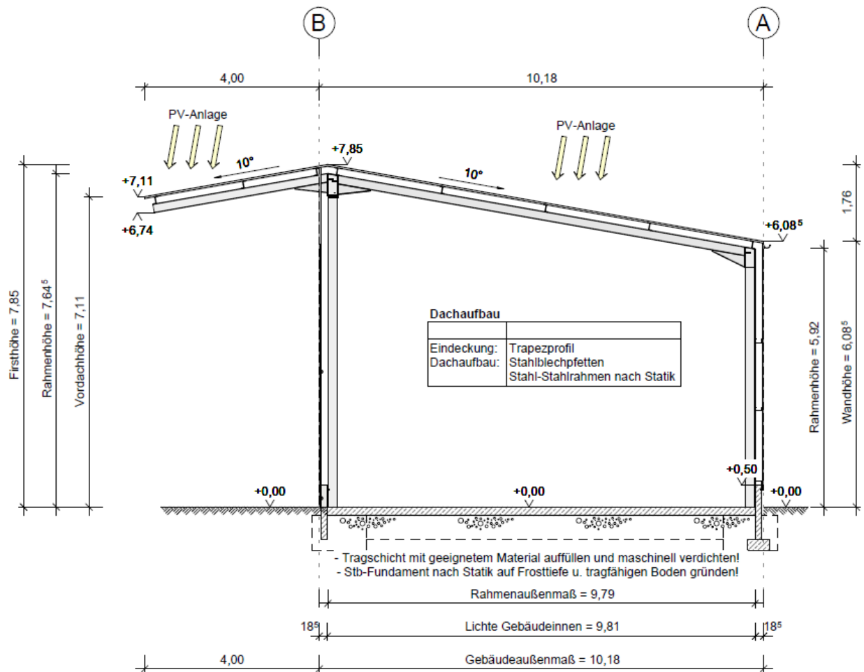
Schnitt A-A
