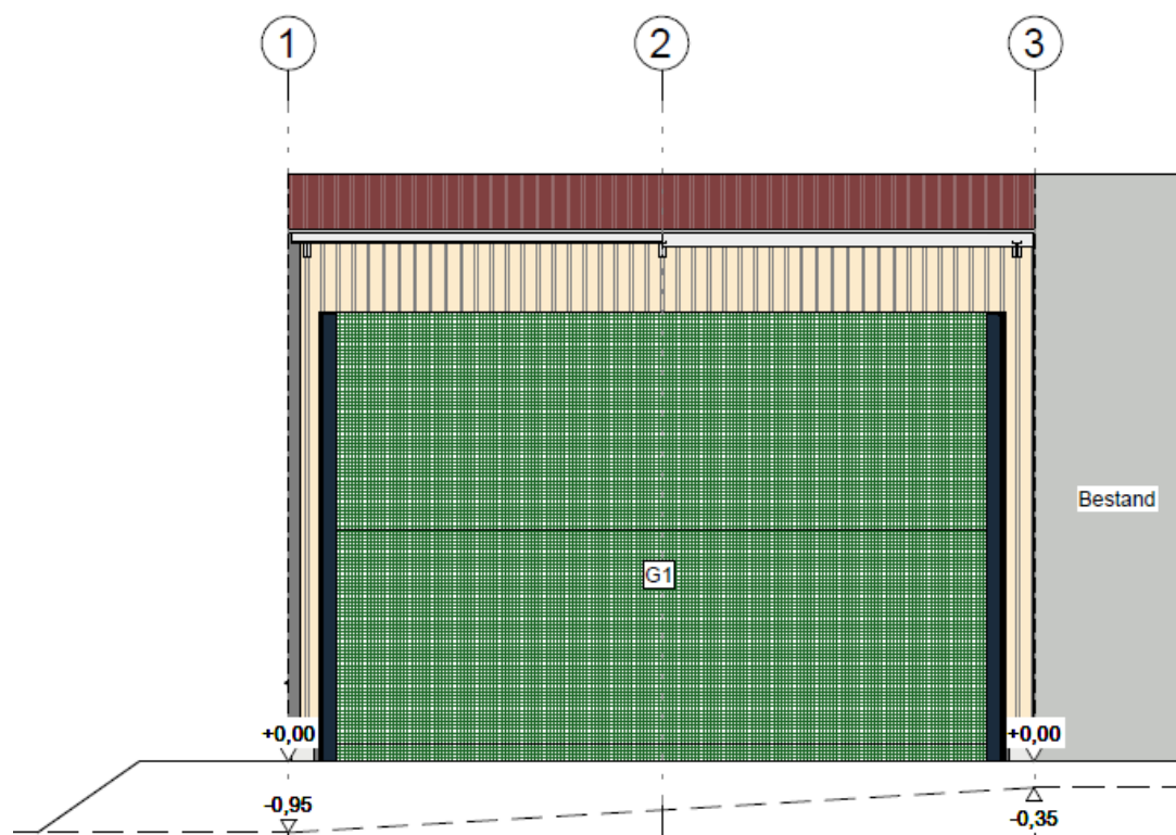
Ansicht Nord-Ost
