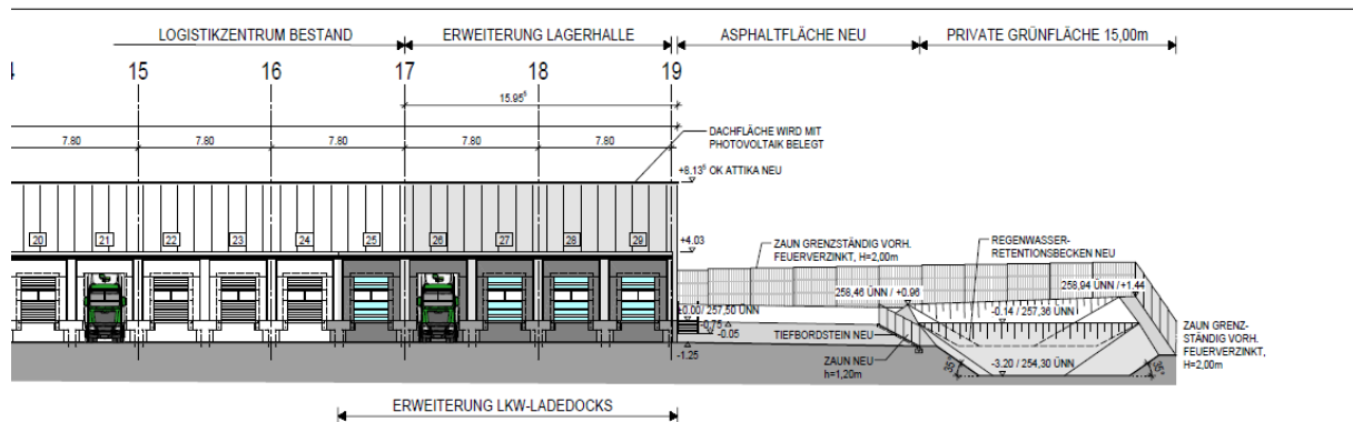
Ansicht Ost
