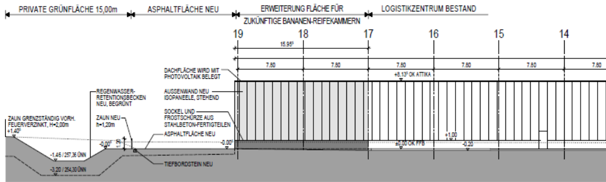
Ansicht West
