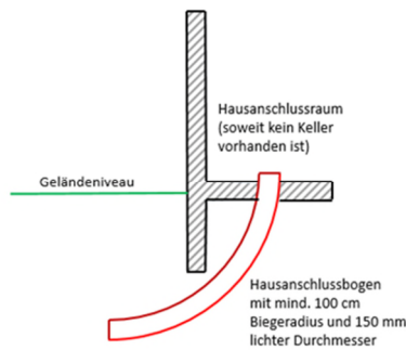
Abbildung 1: Hausanschlussbogen
